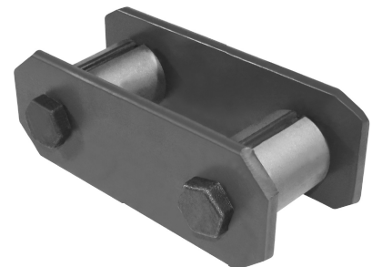
741.702 = JUMELO DA MOLA TRAS. IVECO EUROTECH 450 (COMPLETO)
