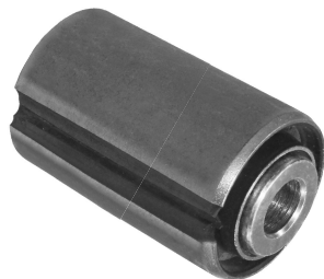
102.703 = BUCHA DO JUMELO TRASEIRA P/ TRASEIRA IVECO EUROTECH 450 N°. ORIG. (7.143.407)
